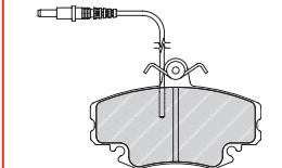
FDB1083 LUC 20961 87 x 53 x 17mm
