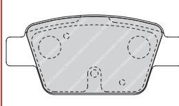
FDB1469 BOS 23714 95 x 42.9 x 15.8mm
