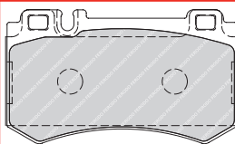
FDB1809 BRE 23478 111.6 x 64 x 15.5mm
