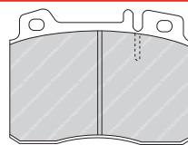
FDB1809 BRE 23478 111.6 x 64 x 15.5mm
