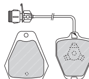
FDB1655 TRW 23326 116 x 59 x 17.5mm
