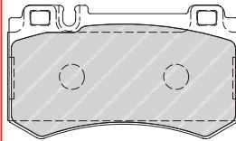
FDB1809 BRE 23478 111.6 x 64 x 15.5mm
