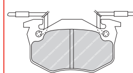
FDB1112 LUC 23124 130 x 56 x 19mm
