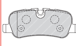
FDB1613 TRW 24192 116.6 x 46.5 x 17.3mm
