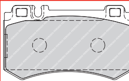
FDB1809 BRE 23478 111.6 x 64 x 15.5mm
