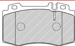
FDB1661 BRE 23745 120 x 71.4 x 17.7mm
