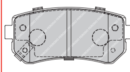
FDB1956 MAN 24320 93.2 x 41.1 x 16mm
