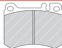
FDB1426 BRE 23271 120 x 71.4 x 17.7mm
