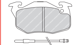
FDB1070 CIT 23161 83 x 75 x 15.3mm
