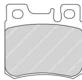
FDB1426 BRE 23271 120 x 71.4 x 17.7mm
