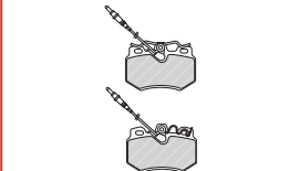
FDB1063 LUC 21674 130 x 57 x 18mm
