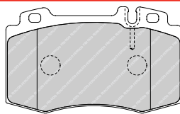
FDB1661 BRE 23745 120 x 71.4 x 17.7mm
