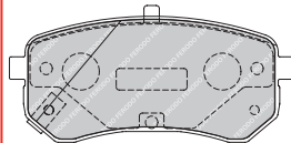
FDB1902 MAN 24276 92.5 x 41 x 14.8mm
