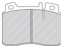
FDB1809 BRE 23478 111.6 x 64 x 15.5mm
