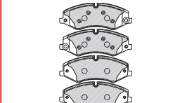
FDB4455 TRW 25021 192 x 72 x 21mm
